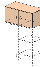
37T015 900x453x430
