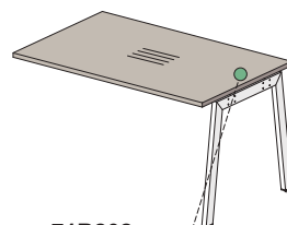
71B202 1326x820x732
