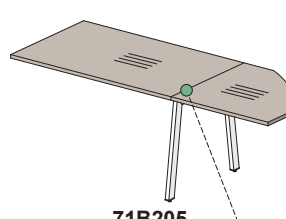
71B205 2175x820x732
