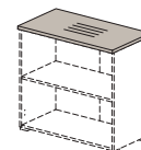
76H0015 786x420x22
