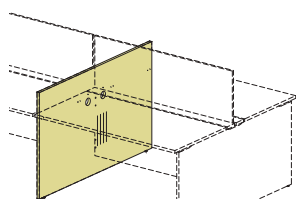
76S3012 1472x22x902
