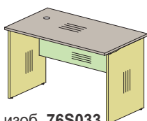
изоб. 76S033 зерк. 76S034 1180x670x737
