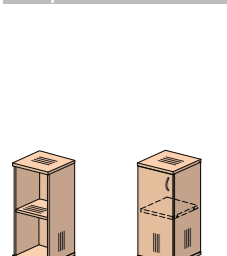
ШС53-04 372X372X800 изоб. ШС52-04L зер. ШС52-04R 372X372X800
