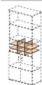
29P003 701X339X334
