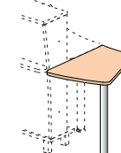
31R044 571x782x739
