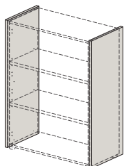
49C002 50*Х450Х1171
