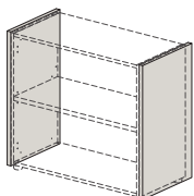
49C001 50*Х450Х787
