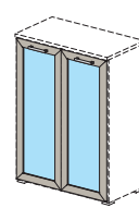
без замка 76H0022 с замком 76H2022 764x16x1022
