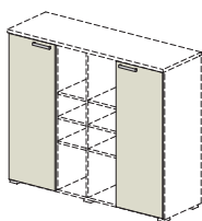
без замка 76H0023 с замком 76H2023 764x16x1022
