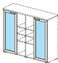
без замка 76H0022 с замком 76H2022 764x16x1022
