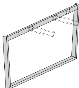
Опора большая
